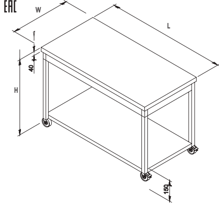
HAREKETLİ TABAN RAFLI ÇALIŞMA TEZGAHI
