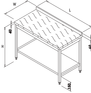
POLİETİLEN TABLALI TABAN RAFLI ÇALIŞMA TEZGAHI
