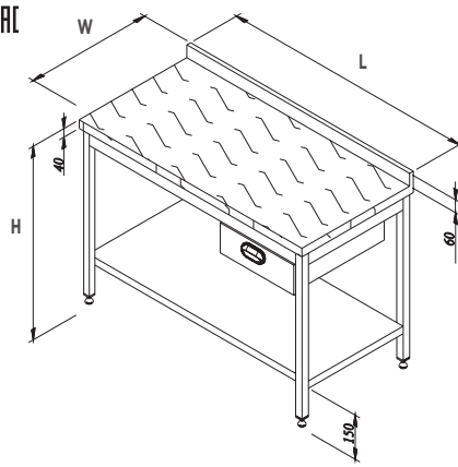
POLİETİLEN TABLALI ÇEKMECELİ, TABAN RAFLI ÇALIŞMA TEZGAHI
