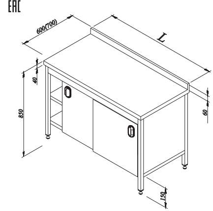
DOLAPLI, ARA RAFLI ÇALIŞMA TEZGAHI
