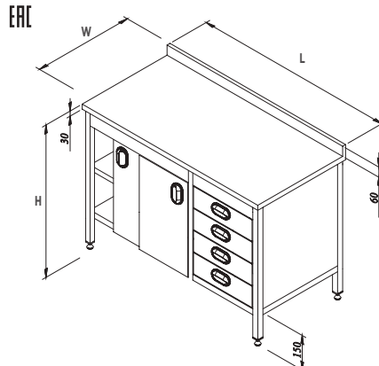
BLOK ÇEKMECELİ ARA RAFLI DOLAPLI ÇALIŞMA TEZGAHI
