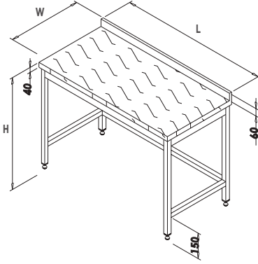
POLİETİLEN TABLALI TABAN RAFSIZ ÇALIŞMA TEZGAHI
