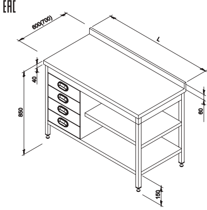
BLOK ÇEKMECELİ, ARA RAFLI ÇALIŞMA TEZGAHI
