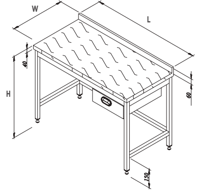
POLİETİLEN TABLALI ÇEKMECELİ, TABAN RAFSIZ ÇALIŞMA TEZGAHI
