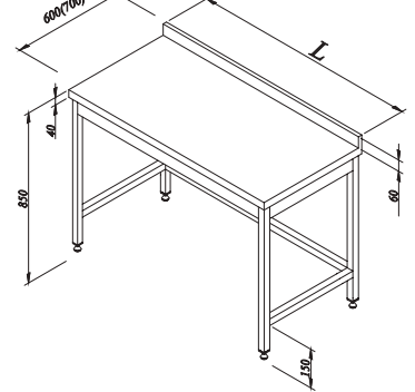
TABAN RAFSIZ, SİRTLİ ÇALIŞMA TEZGAHI
